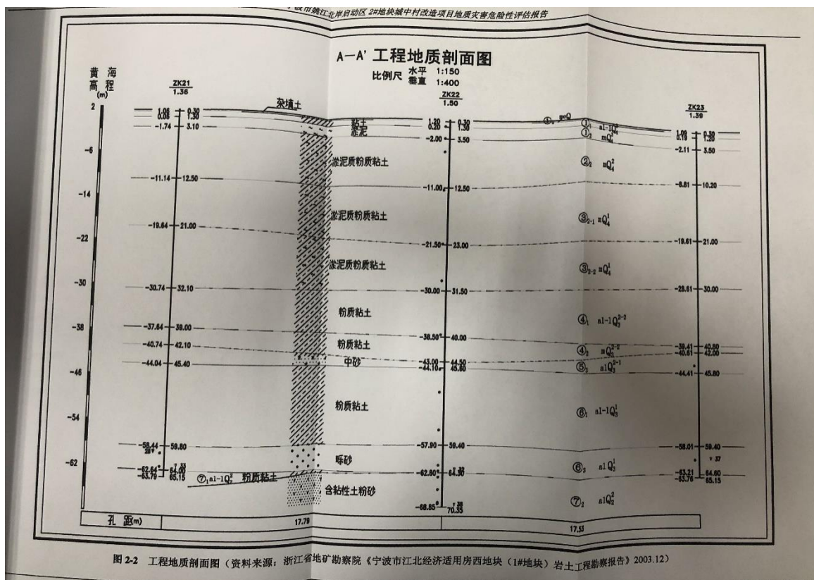
图 2-2 工程地质剖面图
